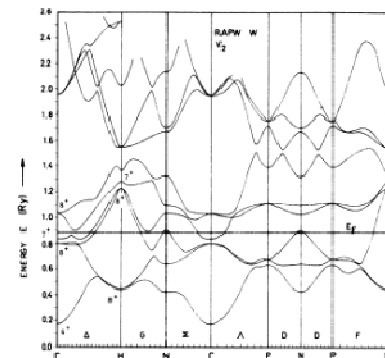
先行論文によるタングステン単結晶のバンド計算
