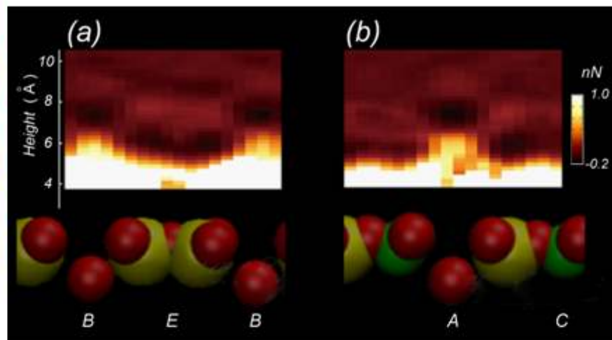
マイカ表面に垂直な面の各位置で探針モデルが感じる力を可視化した図[M. Tsukada, et al., J. Vac. Sci. Technol. B 28, C4C1 (2010)]
