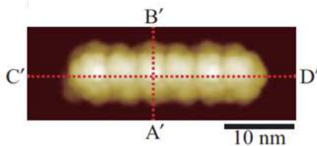
GeoAFMシミュレーション画像
