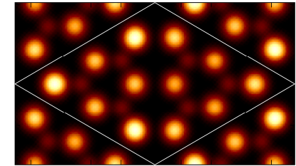
Si(111)7x7DAS構造のDFTBシミュレーション結果
