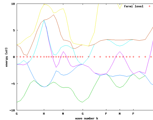
最適化された軌道によるタングステン単結晶のバンド計算の結果
