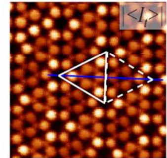
Si(111)7x7DAS構造のDFTBシミュレーション結果
