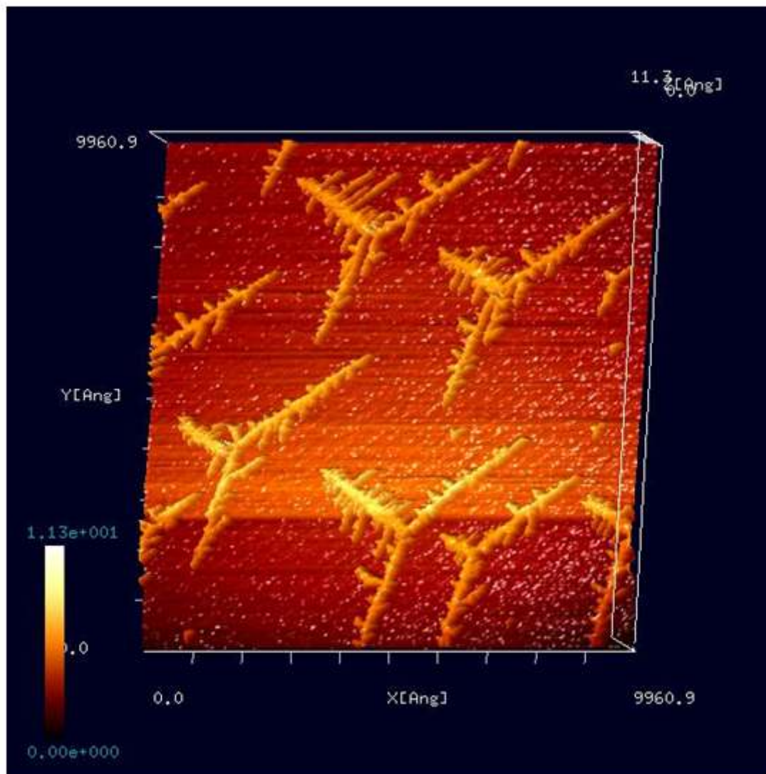
Analyzer:実験画像表示機能(Ir結晶表面上に蒸着されたAuのフラクタル島状構造)
